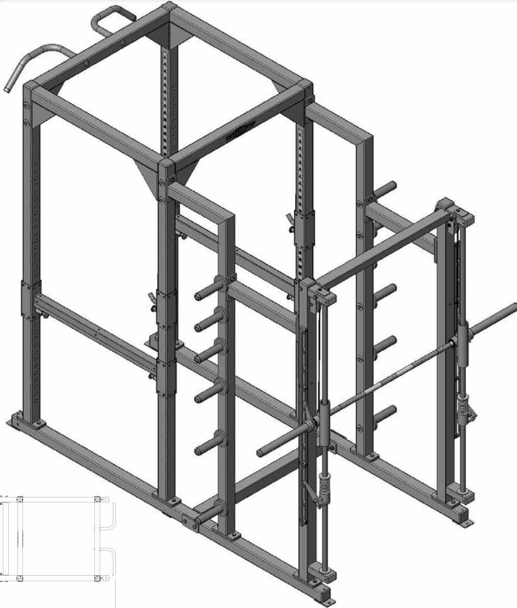
XXL-2960 L 112" W 86" H 100"
